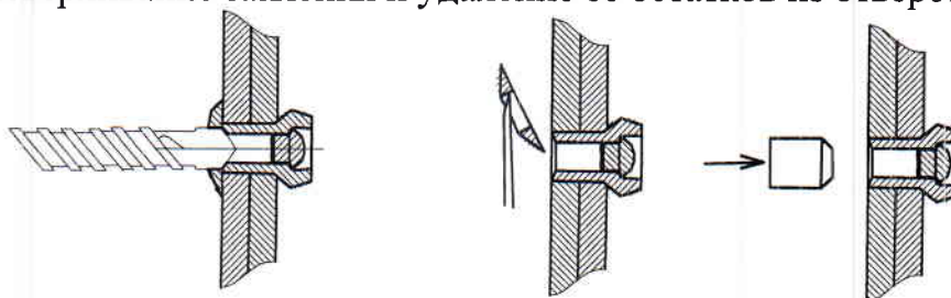
Рис. 11. Удаление заклепки
