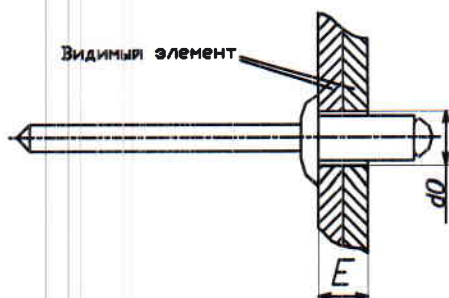
Рис. 6. Геометрические параметры соединяемых элементов
