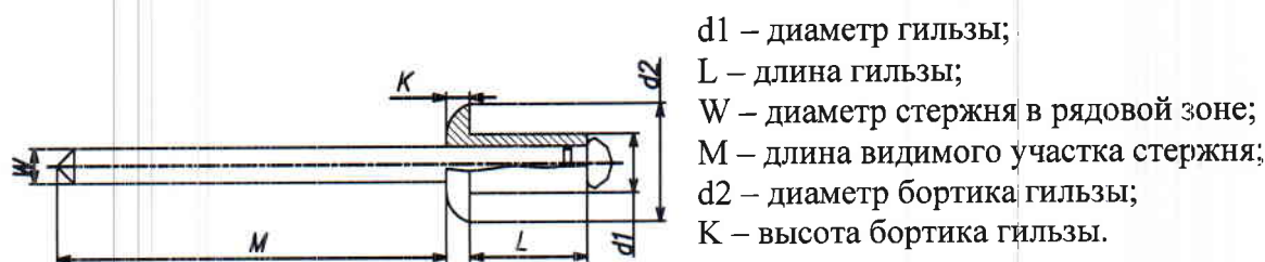
Рис. 3. Основные геометрические параметры заклепки до установки в проектное положение
