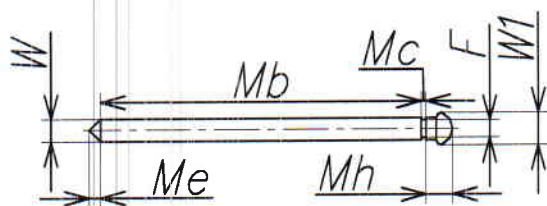
Рис. 5. Геометрические параметры стержня
