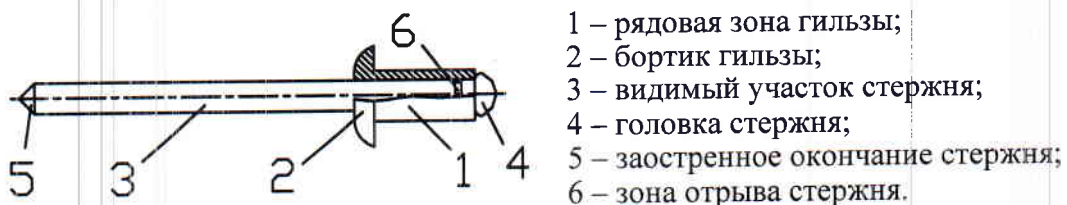
Рис. 1. Общий вид заклепки
