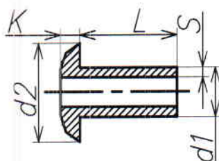
Рис. 4. Геометрические параметры гильзы
